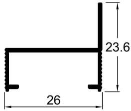
CM060 0,276 Kg/m Requadro em alumínio natural
