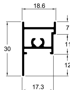
MH138 0,310 Kg/m Folha travessa superior com baguete
