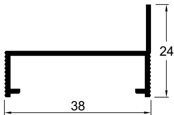
CM174 0,409 Kg/m Requadro em alumínio natural
