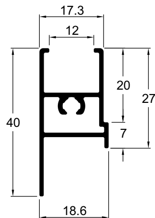
MH099 0,374 Kg/m Folha travessa inferior sem baguete
