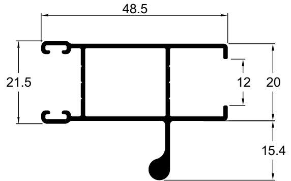
MH056 0,572 Kg/m Folha montante lateral com reforço
