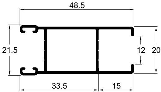
MH055 0,461 Kg/m Folha montante lateral
