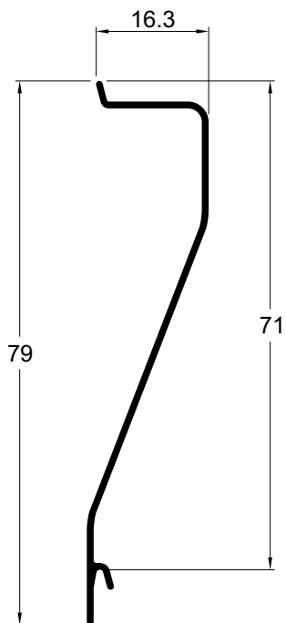
VZ072 0,260 Kg/m Palheta veneziana cega
