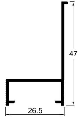
CM098 0,387 Kg/m Travessa inferior do requadro para porta
