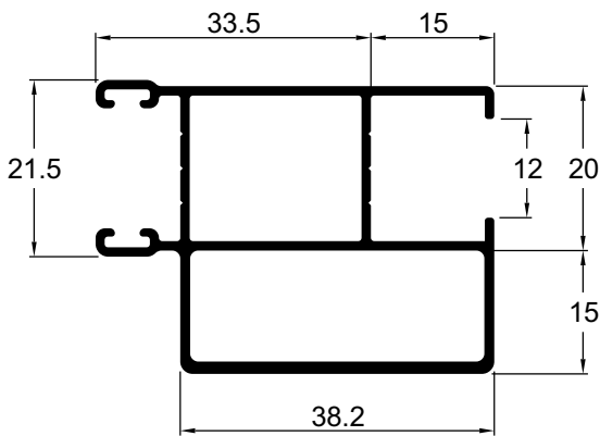
MH063 0,900 Kg/m Folha montante lateral com reforço
