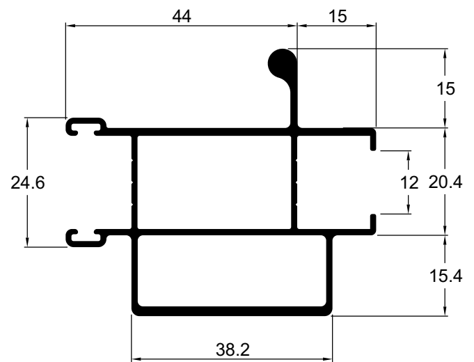
MH205 0,973 Kg/m Folha montante lateral com reforço duplo
