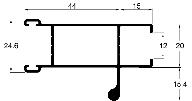
MH204 0,639 Kg/m Folha montante lateral com reforço para fechadura
