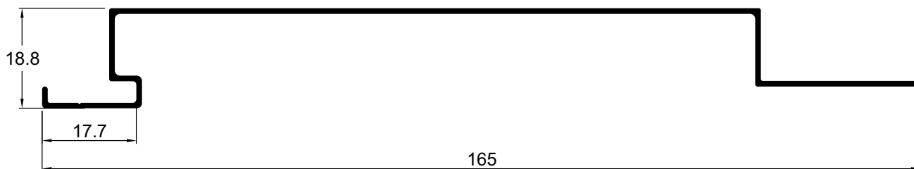
LU083 0,839 kg/m
