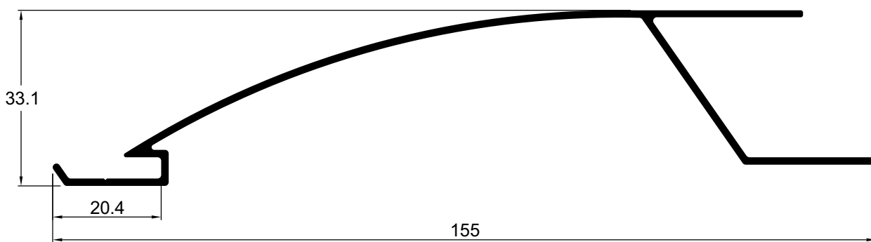
LB089 0,581 kg/m
