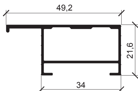
ADR 230 Premarco 0,463 kg/m
