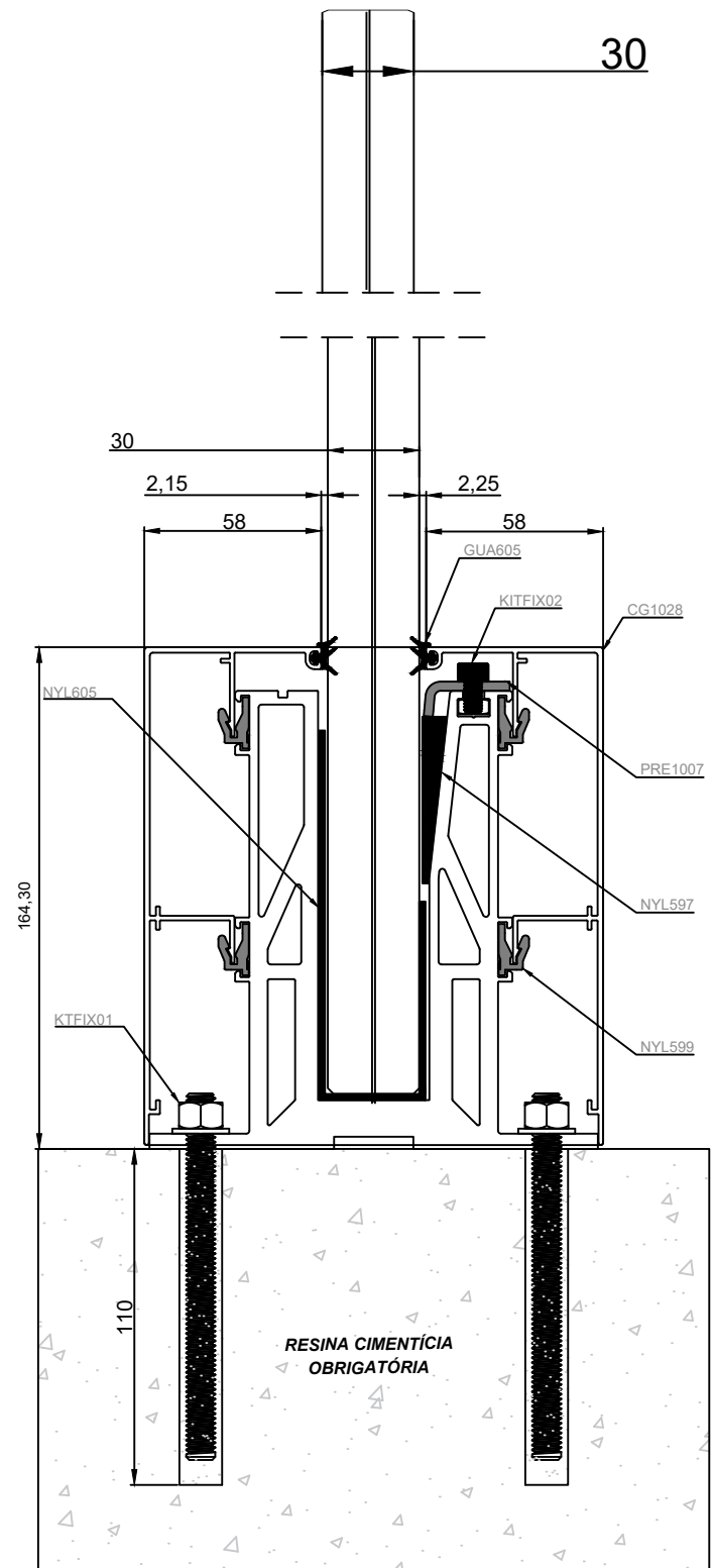
Detalhamento KITGR12 com vidros de 30mm
