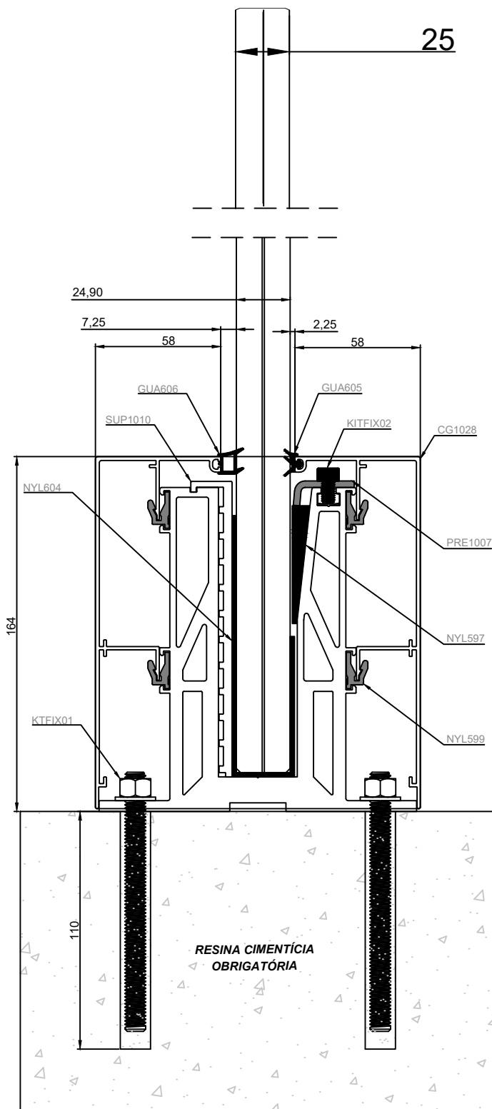
Detalhamento KITGR12 com vidros de 25mm
